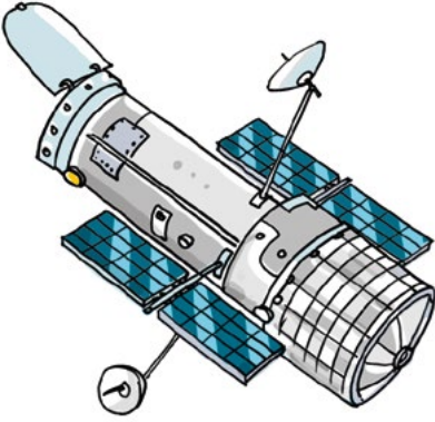
Uzay teleskobı
