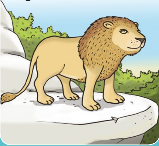
Mağara aslanı
