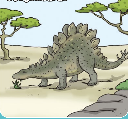
Stegosaurus
